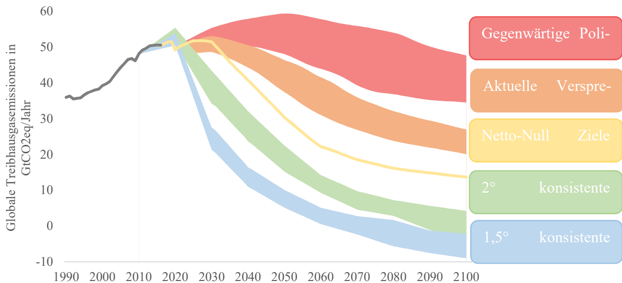
Abb. 2: Globale jährliche Treibhausgasemissionen und Erderwärmungsprognosen verschiedener Szenarien bis 2100, Stand Dezember 2020. Quelle: Eigene Darstellung in Anlehnung an Climate Action Tracker (Hrsg.) (2020), 2100 warming projections.
